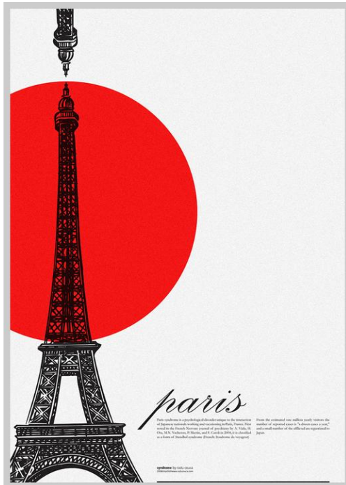
Gambar 3.13 Kontras meskipun sederhana tetap berperan sebagai stopping power
